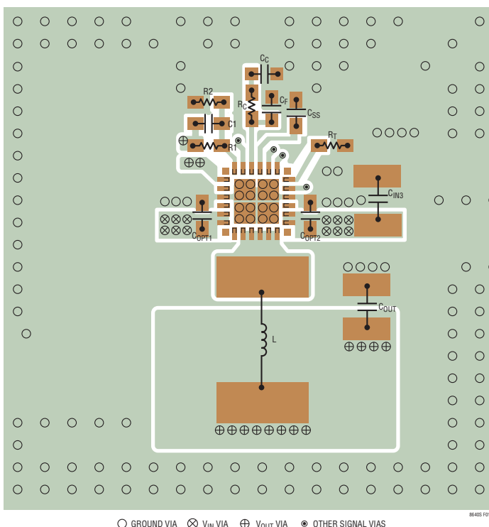
(b) LT8643S/LT8643SA
