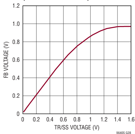
Soft-Start Tracking (LT8643S/LT8643SA)
